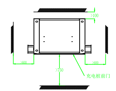
充电桩四周与障碍物距离尺寸示意图
