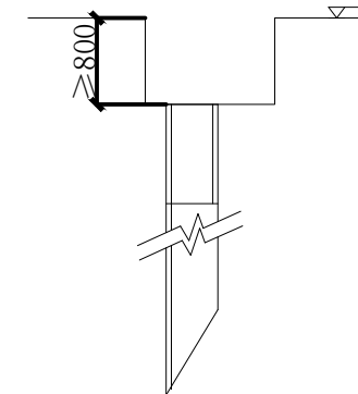
接地体入地示意图
