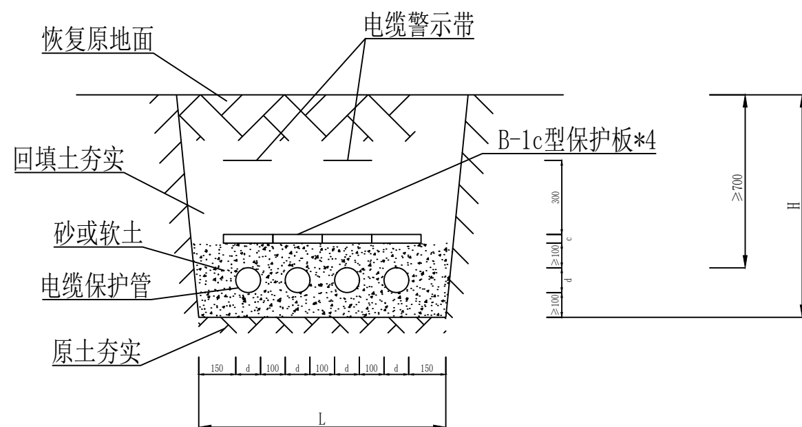
4根电缆并列敷设
