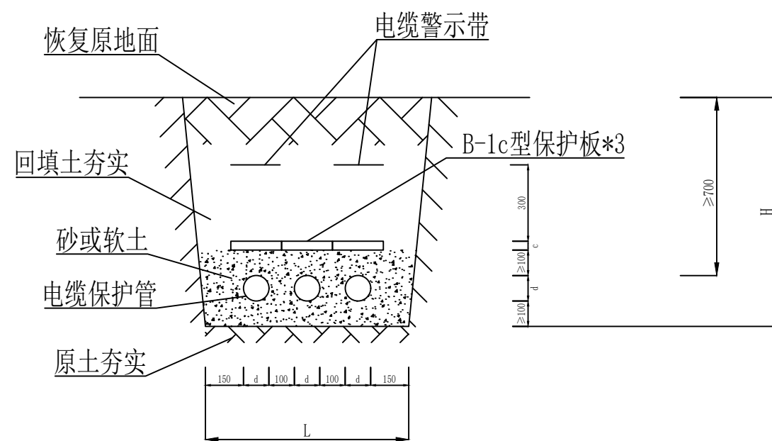
3根电缆并列敷设
