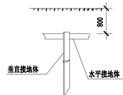
接地体的埋入深度
