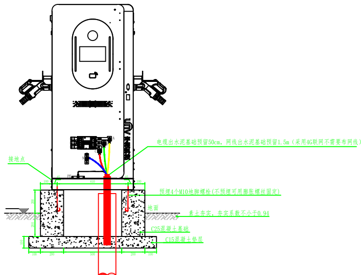
剖面图1
