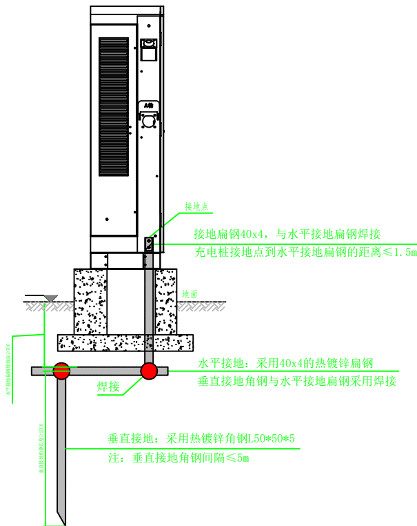
接地示意图
