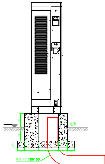
剖面图2
