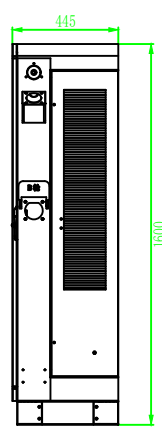
右视图
