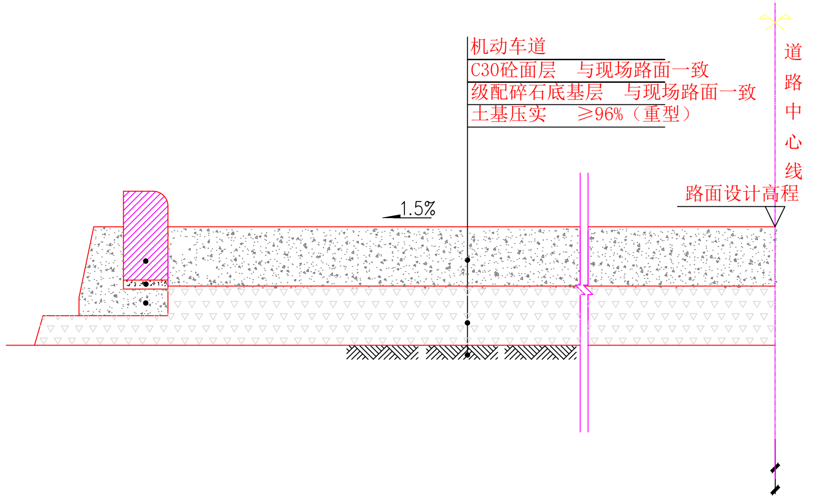
道路结构图
