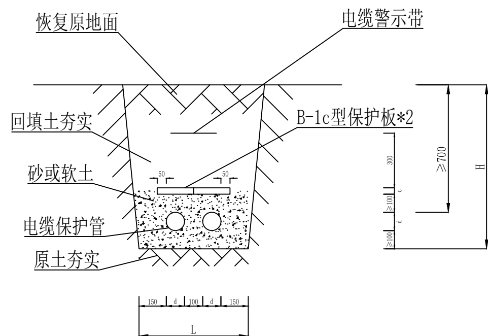
2根电缆并列敷设
