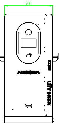
主视图
