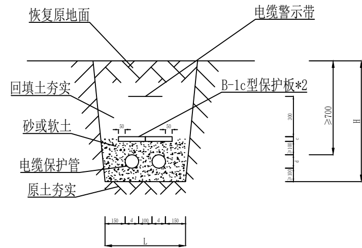
2根电缆并列敷设
