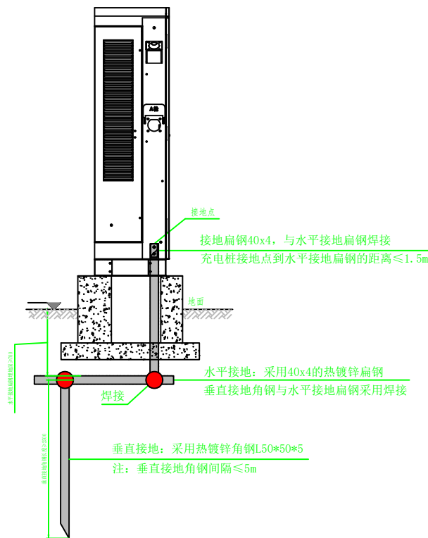
接地示意图
