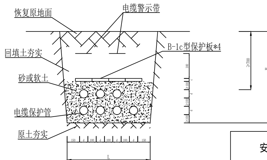
7根电缆双排敷设
