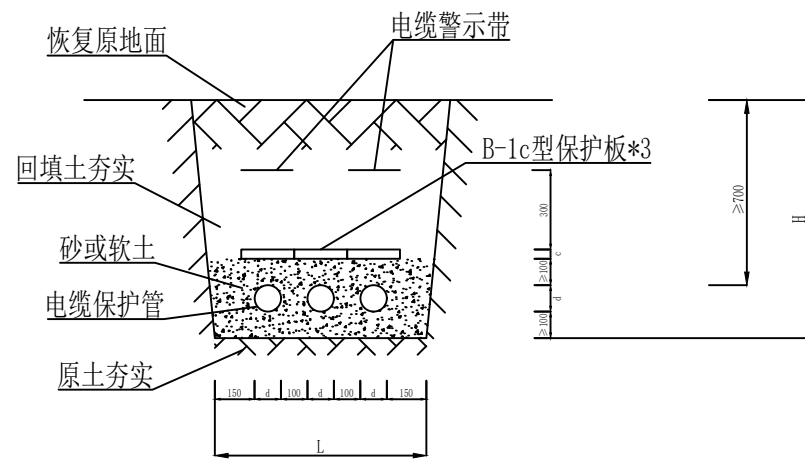
3根电缆并列敷设
