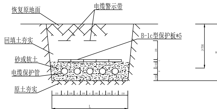
5根电缆并列敷设
