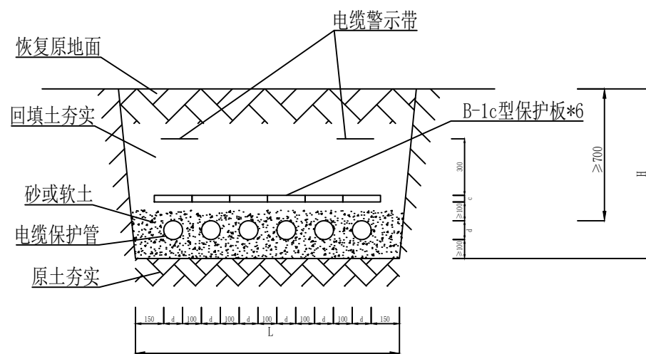
6根电缆并列敷设
