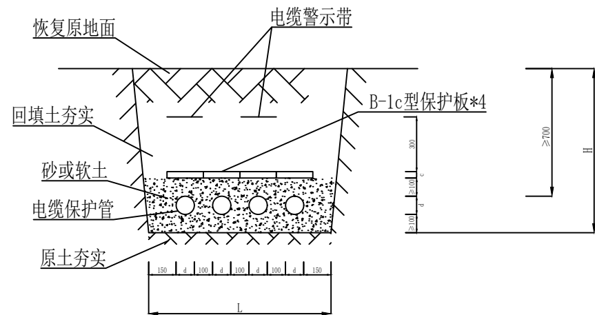
4根电缆并列敷设
